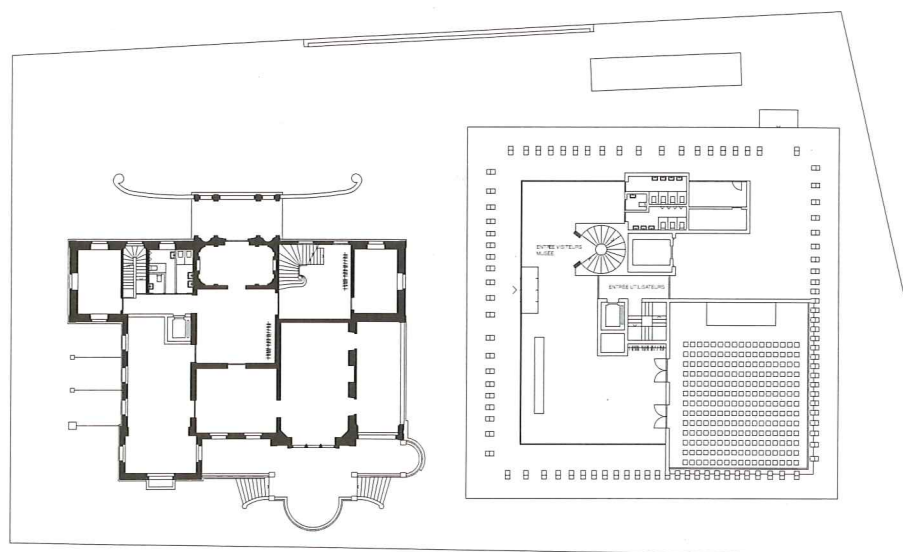
Grundriss EG
