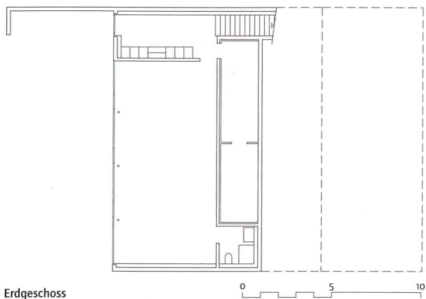
Erdgeschoss
